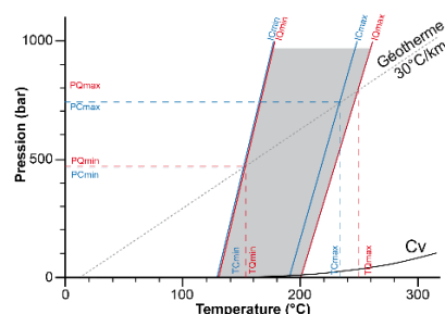
Figure 1 : Synthèse des isochores calculées
